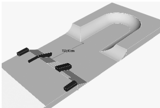
Komputerowa wizualizacja projektu skateparku.
